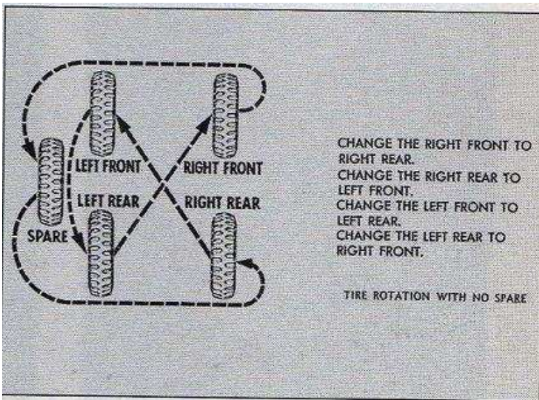
Rotation des pneumatiques avec et sans roue de secours pour Dodge
